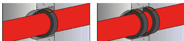
Enkel tätning < \varnothing 75 mm
