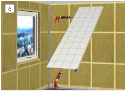
6 Påför godkänd fogmassa på sågade ytor. Se bild. Dra ut fogmassan med fogkloss.
